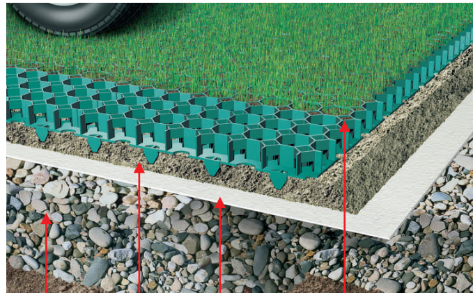
zhuťný štěrk písek geotextilie GUTTATEX zemina
