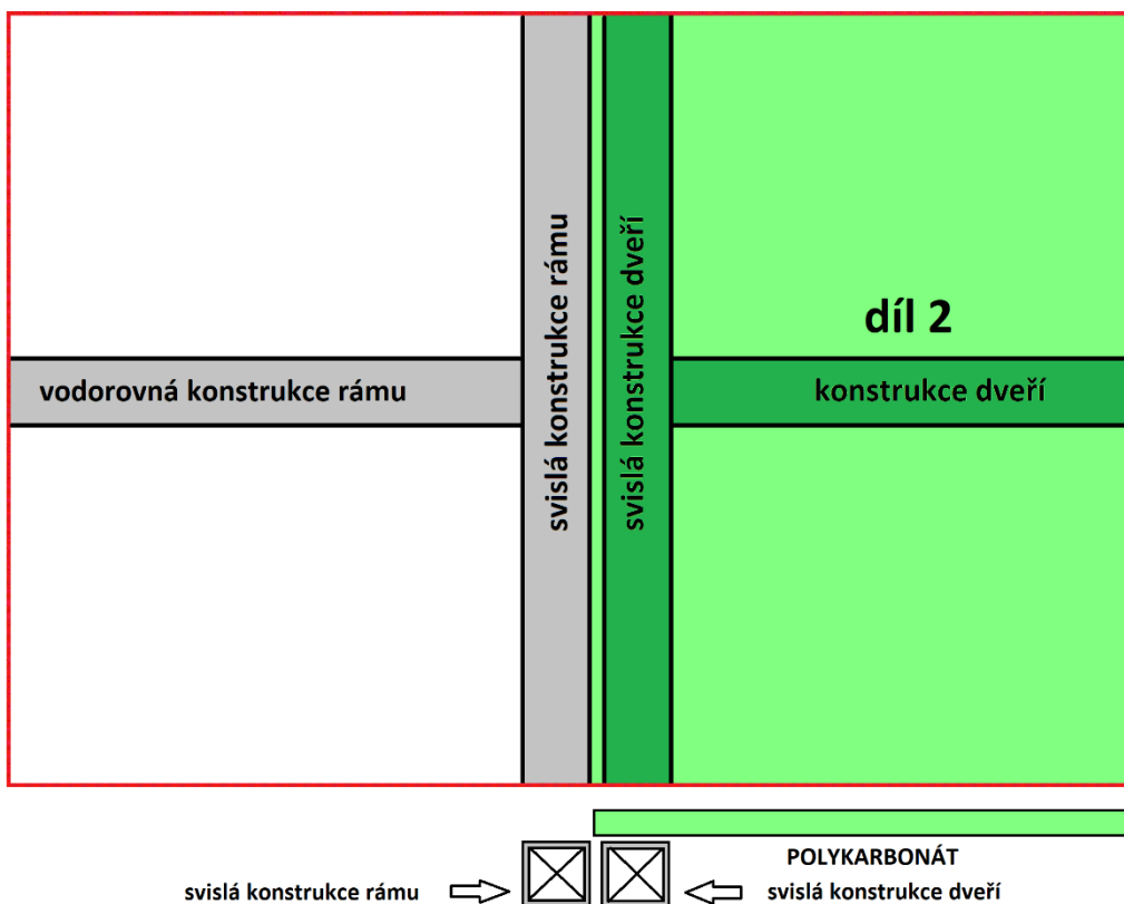
Obr. 2 – díl 2 posuňte až ke kraji svislé konstrukce rámu dveří (přes okraj konstrukce dveří)
